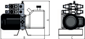
Montaggio orizzontale Horizontal mounting
